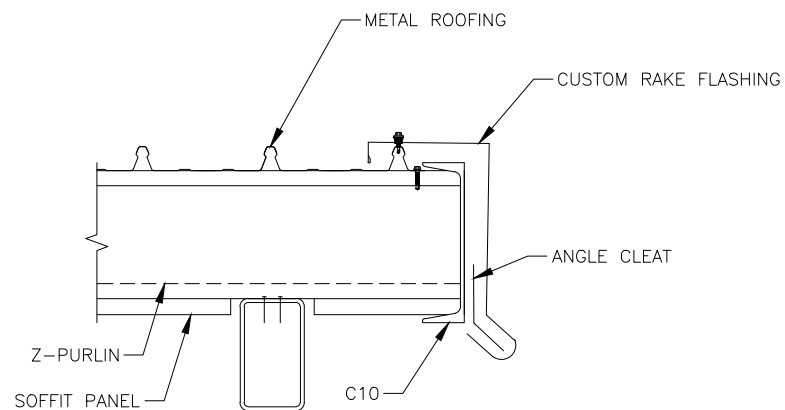
5 RAKE ON MODULE Z PURLIN -- 1"=1'-0"
