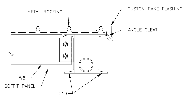
2 RAKE ON MODULE W SECTION -- 1"=1'-0"
