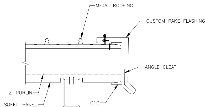
4 RAKE OFF MODULE Z PURLIN -- 1"=1'-0"
